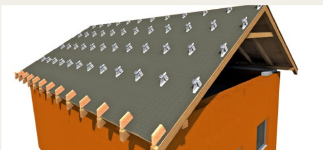
4. Montáž kovových držáků a ukončovacích dřevěných hranolků Kovové držáky jsou kotveny pomocí speciálních pozinkovaných hřebů odolných proti vytržení. Pro kotvení 1 ks kovového držáku je nutné použít 4 hřebů délky 40 mm a 6 hřebů délky 60 mm. Délka 40 mm je určena do přídavné krokve, délka 60 mm je určena do krokve (paty držáku).
