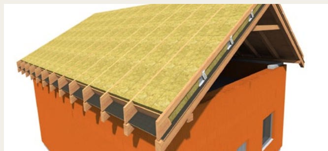
6. Pokládka 2. vrstvy izolace mezi pomocné krokve v tloušťce odpovídající výšce pomocné krokve: – 80 až 120 mm v případě použití kovového držáku 120 mm – 60 až 120 mm v případě použití kovového držáku 180 mm
