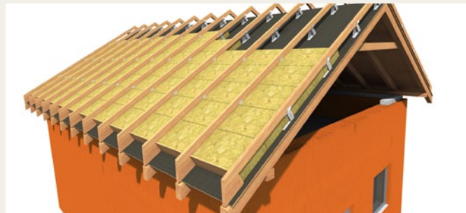
5. Montáž pomocných krokví 60 × 60 až 120 mm a vložení první vrstvy izolace ROCKMIN PLUS , SUPERROCK nebo ROCKTON v tloušťce odpovídající výšce kovového držáku: 120 mm nebo 180 mm.
